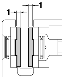
1. Limite d'usure de plaquette de frein de stationnement
