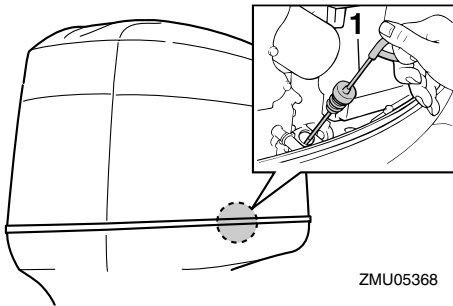
1. Jauge d'huile
