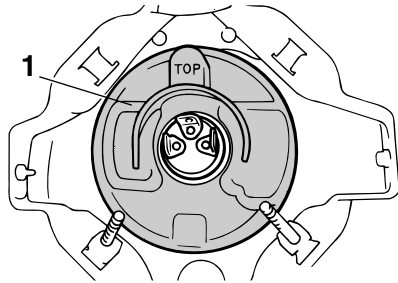
1. Protection d'ampoule
