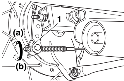
1. Écrou de réglage de la garde de la pédale de frein
