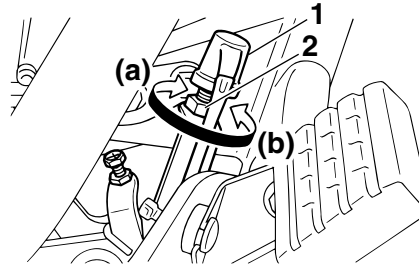
1. Écrou de réglage de la garde de la pédale de frein
