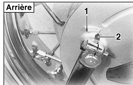
1. Trait d'indication de limite d'usure 2. Index d'indication d'usure des mâchoires de frein
