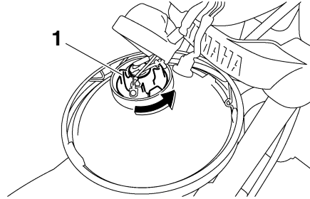
1. Douille d'ampoule de phare
