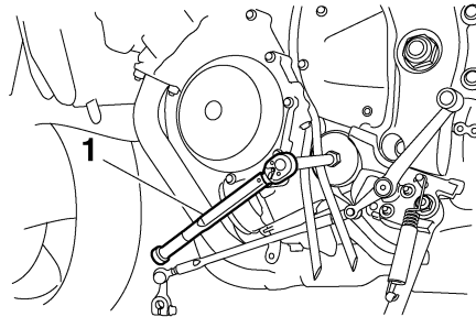
1. Clé dynamométrique
