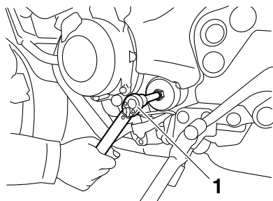
1. Clé dynamométrique
