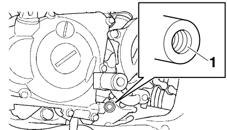
1. Orifice de la vis de contrôle du niveau d'huile moteur
