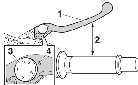
1. Maneta de freno 2. Distancia entre la maneta del freno y el puño del acelerador 3. Dial de ajuste de la posición de la maneta de freno 4. Marca “ \Delta ”
