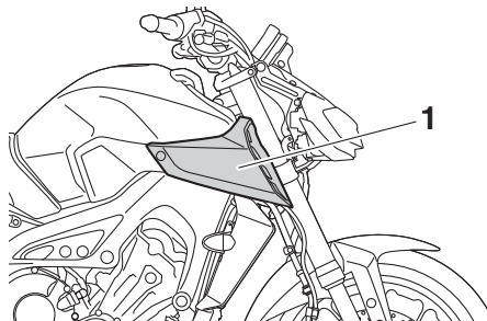
1. Cache A
