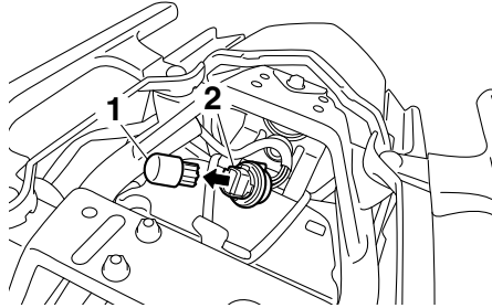
1. Ampoule de feu arrière/stop 2. Douille d'ampoule de feu arrière/stop
