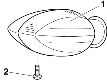
1. Lentille du clignotant 2. Vis
