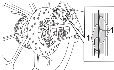
1. Rainure d'indication d'usure
