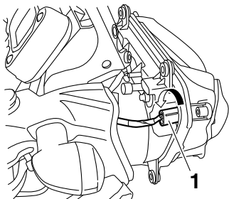
1. Douille d'ampoule de veilleuse
