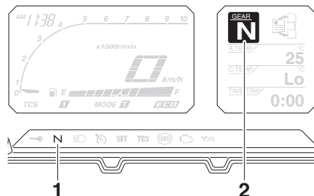
1. Témoin du point mort “N” 2. Afficheur du rapport engagé
