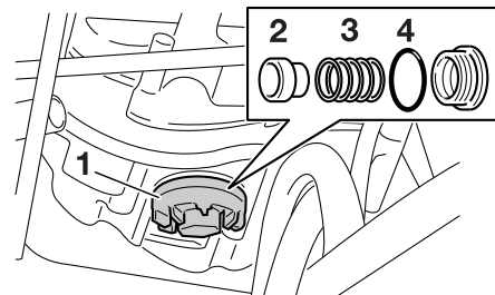
1. Vis de vidange d'huile moteur B 2. Crépine 3. Ressort de pression 4. Joint torique
