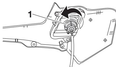
1. Douille d'ampoule de clignotant
